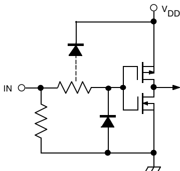
Dwg. EP-010-4A
